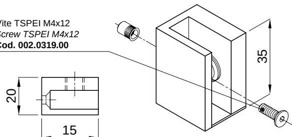
Blocchetto chiuso per fiss. vetro Complete closed glass support
