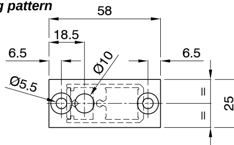
Schema fori di fissaggio Fixing drilling pattern
