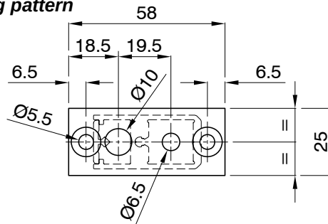
Schema fori di fissaggio Fixing drilling pattern
