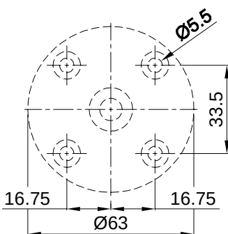
Schema posizione fori di fissaggio Fixing holes layout
