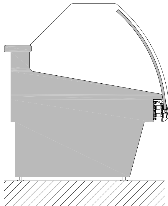
Installazione inferiore del sistema System's lower installation
