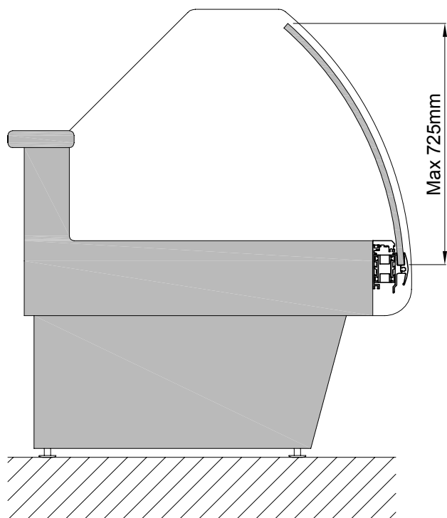
Installazione frontale del sistema System's front installation
