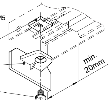
Kit tappo plafoniera completo Complete light canopy end cap kit
