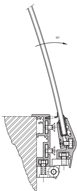
Vetro inclinato 10,5° - R1016 R1016 - 10.5° angle glass
