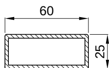
Profilo montante laterale Lateral upright profile
