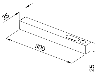
Piede laterale Lateral base plate
