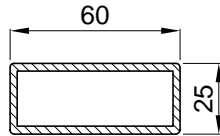
Profilo montante laterale Lateral upright profile
