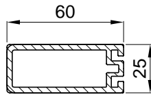
Profilo montante laterale Lateral upright profile
