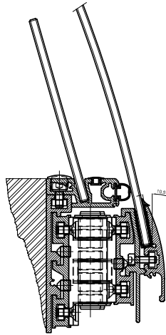
Vetro inclinato 10.5° - R1016
