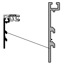
Vetro inclinato 10.5° - R1016
