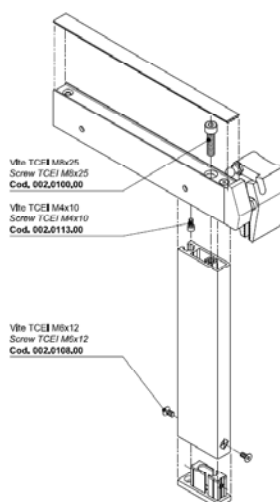
Kit minuteria fissaggio scatola al montante 080 Cod. 001.0521.00 Kit small parts for fixing case to 080 upright
