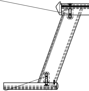
Tirante inferiore Lower tie rod
