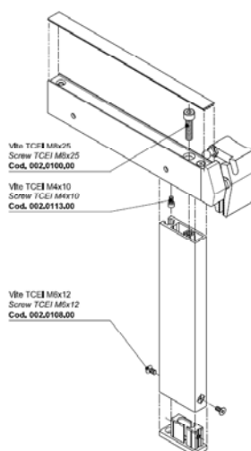
Kit minuteria fissaggio scatola al montante 080 Cod. 001.00521.00 Kit small parts for fixing case to 080 upright
